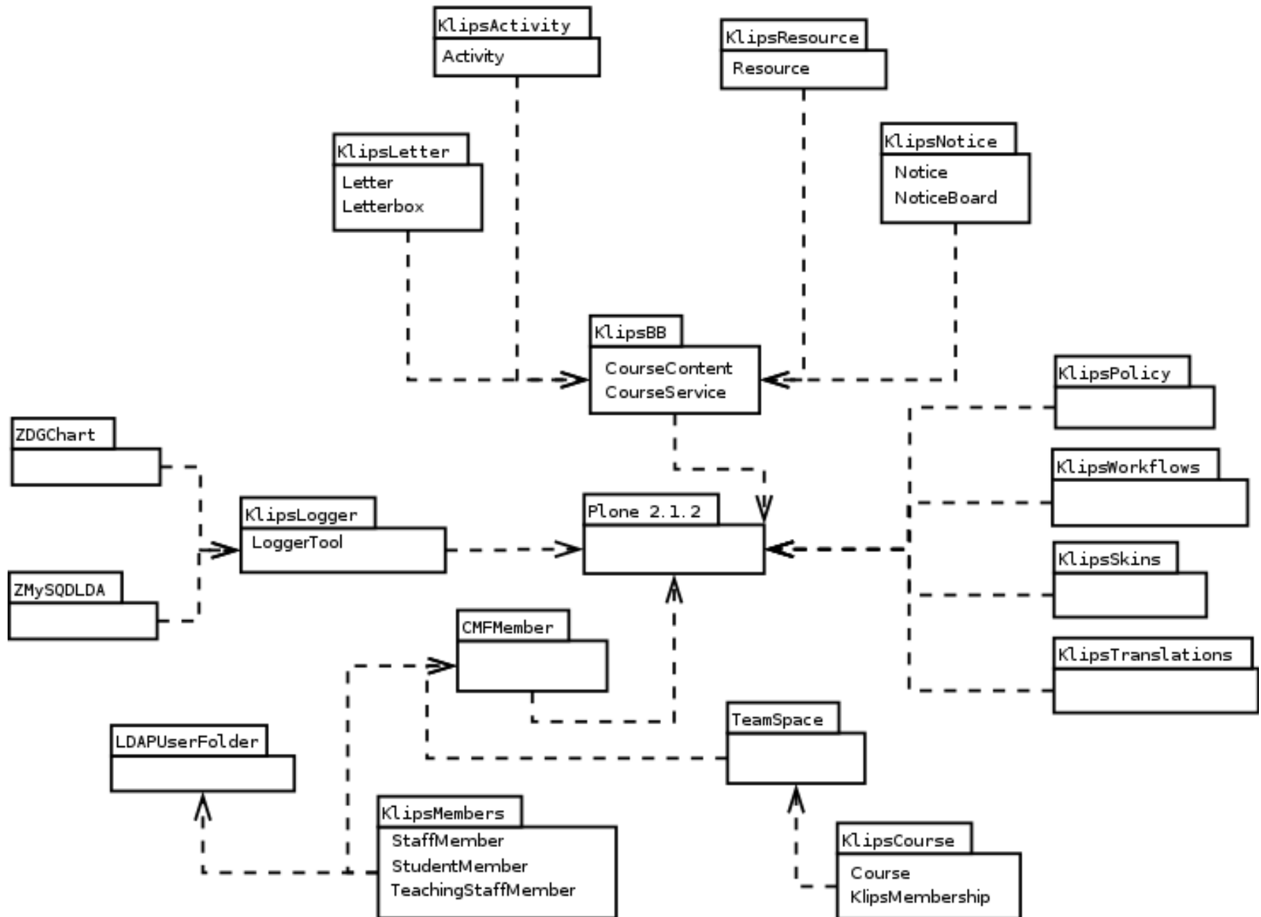
Diagramma delle dipendenze tra i prodotti
